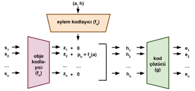
Şekil 2: Eylem ve nesne kodlayıcılı ve ikili darboğaz katmanlı primitif bulma modeli. Nesne kodlayıcısı ( f_o ), nesne s_i ’leri ikili gösterim olan z_i ’lere, eylem kodlayıcısı ( f_a ) da verilen eylem parametresi a ’yı ikili gösterim olan p_h ’ye dönüştürür. p_h yalnızca hedef ( h ) nesne gösterimine ( z_h ) eklenir ve oluşturulan vektörden kod çözücü ( g ) her nesne için etki e_i ’yi tahmin eder.
