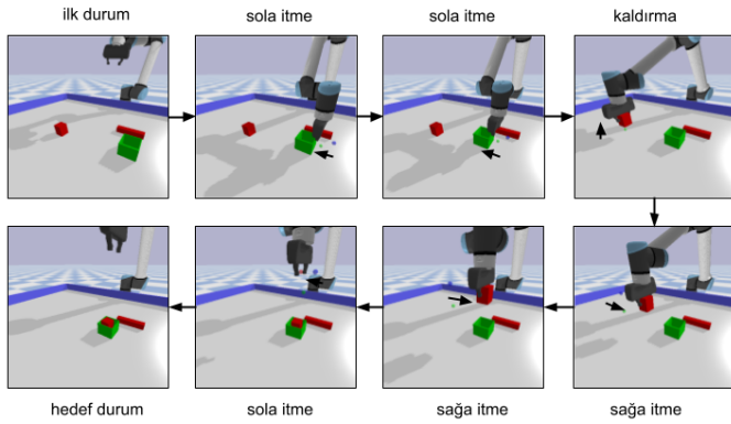
Şekil 5: İlk durumdan hedef duruma götüren 6 adımlı eylem dizisi.
