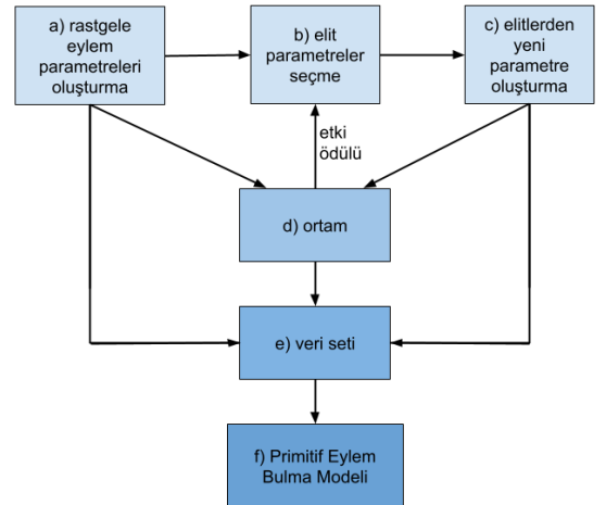
Şekil 3: Aktif Öğrenme Modülü (AÖM). a, b, c, d; robotun ortamı keşfini, e; bu keşiften oluşturulan veri setini, f de bu veri ile eğitilen primitif eylem bulma modelini gösterir.
